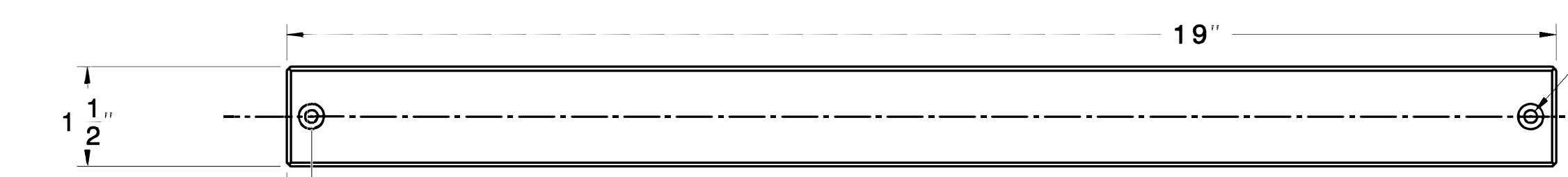
Back Slat view Scale: 1:2
