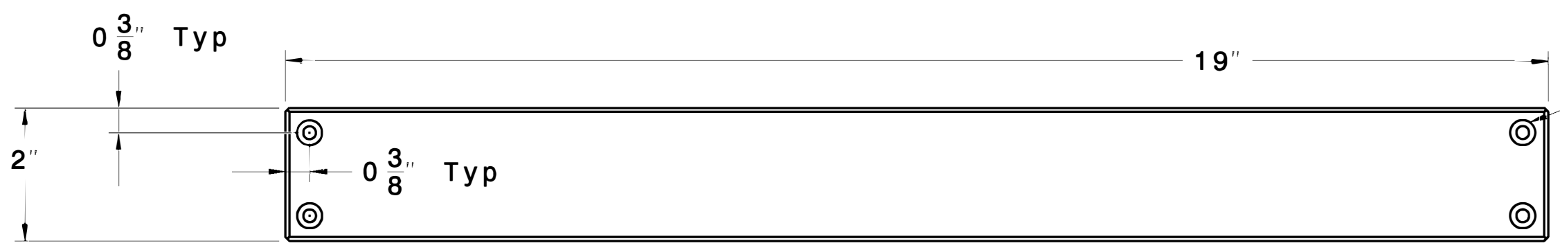
Back Cleat view Scale: 1:2
