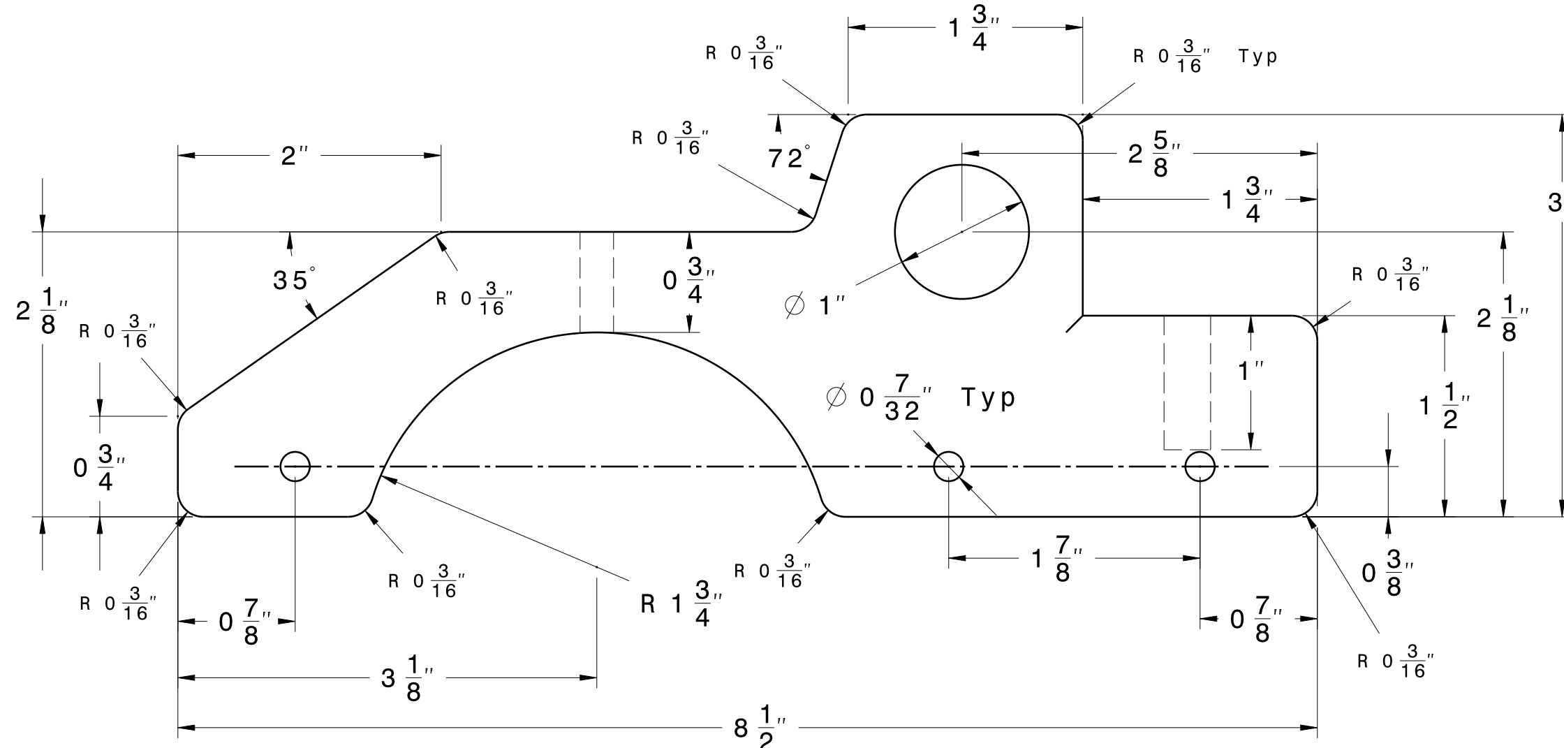
Body Scale: 1:1
