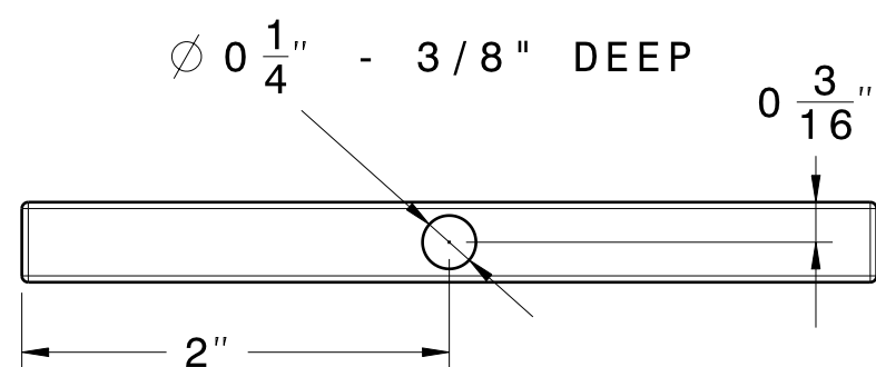
Blade Top view Scale: 1:1
