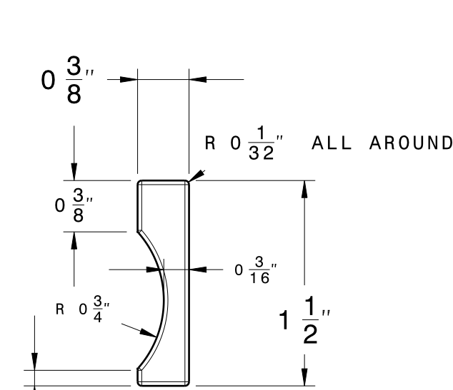
Blade Side view Scale: 1:1
