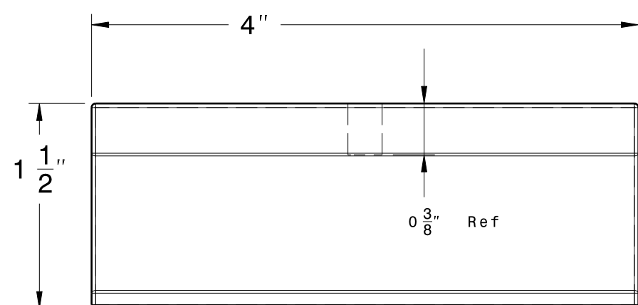
Blade Scale: 1:1
