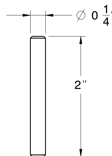
Blade Pivot Shaft Scale: 1:1
