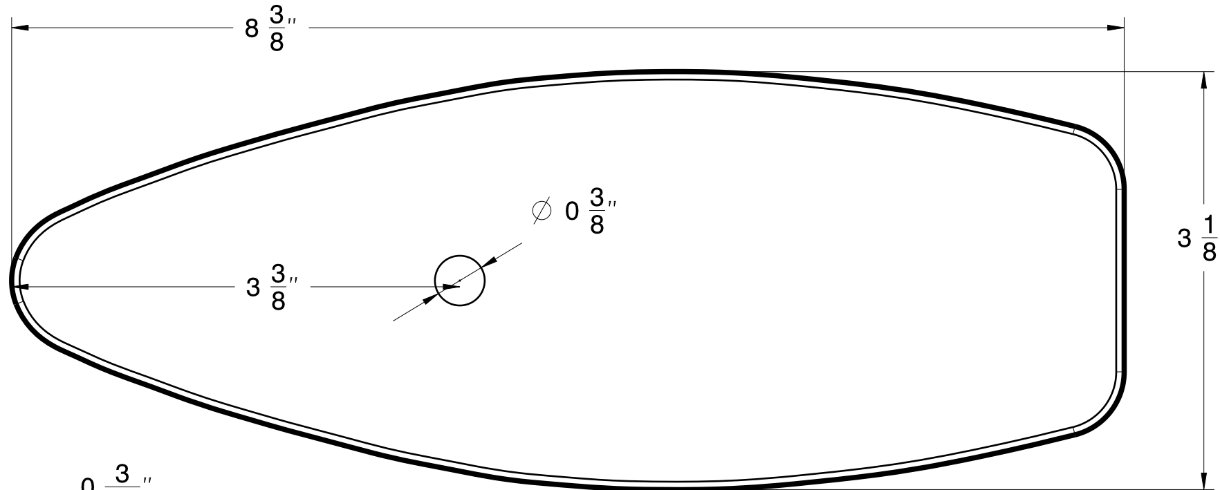
Hull Top view Scale: 1:1
